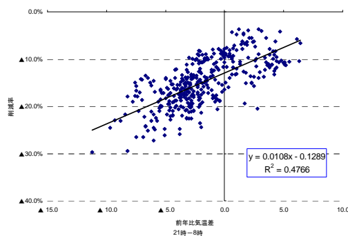
図3-12 気温差と削減率の相関（21-8時） （8月）
