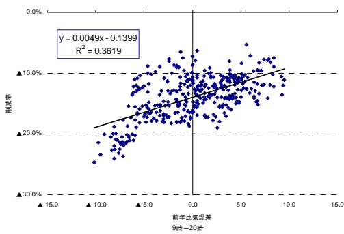
図3-7 気温差と削減率の相関 (9-20時) (6月)
