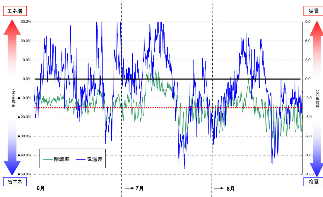
図2-2 対前年気温差と電力需要の削減率（東北電力管内）（6月-8月末）
