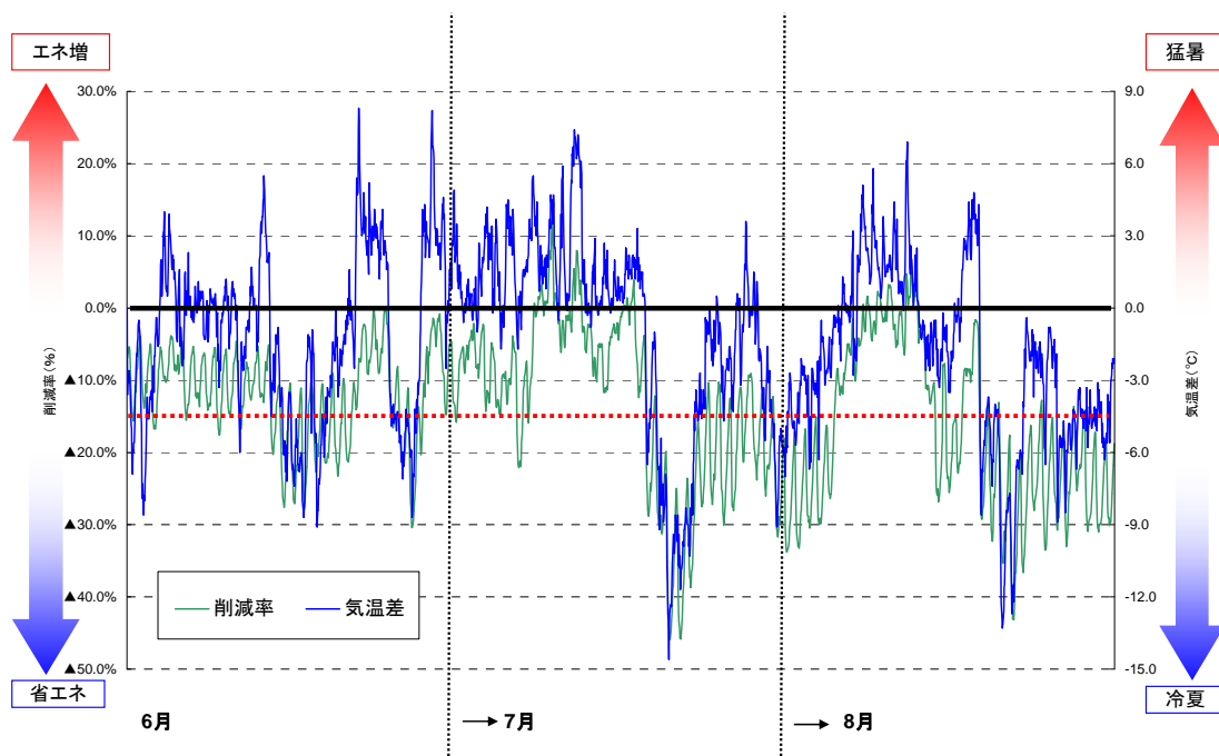
図2-1 対前年気温差と電力需要の削減率（東京電力管内）（6月-8月末）
