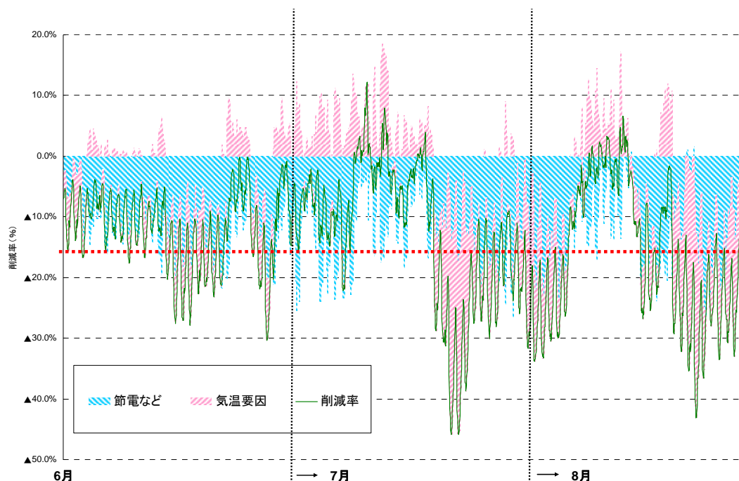
図4-1 要因分解(東京電力管内) (6月-8月末)
