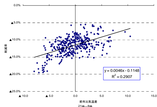
図3-8 気温差と削減率の相関 (21-8時) (6月)
