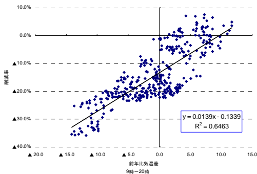
図3-11 気温差と削減率の相関（9-20時） （8月）
