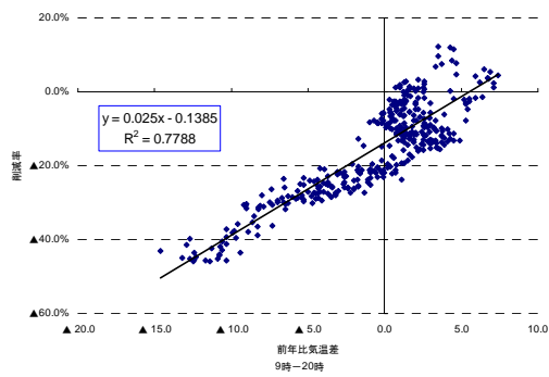
図3-5 気温差と削減率の相関 (9-20時) (8月)
