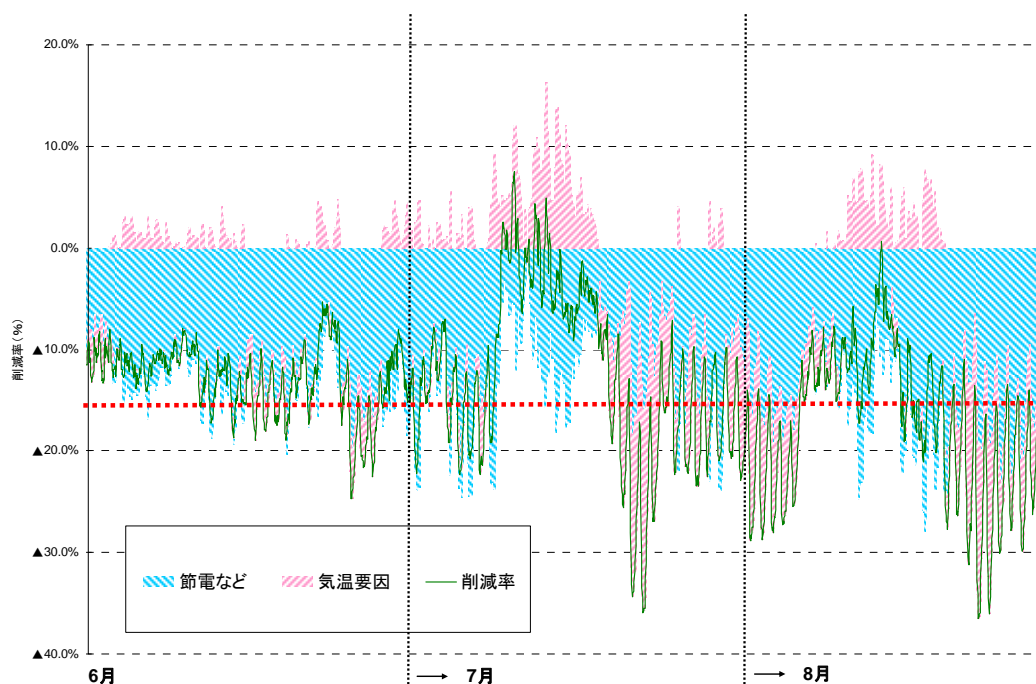
図4-2 要因分解(東北電力管内) (6月-8月末)
