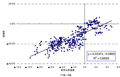
図3-6 気温差と削減率の相関 (21-8時) (8月)
